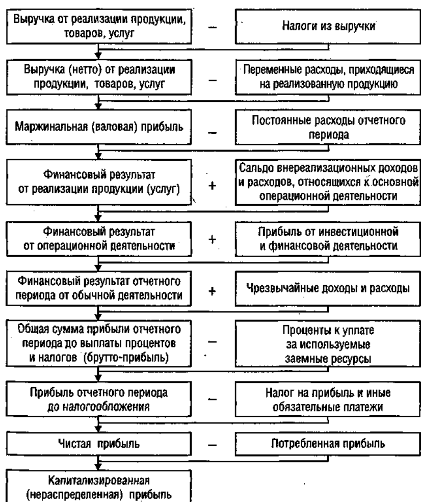
Рис. 8.2. Структурно-логическая модель формирования показателей прибыли
